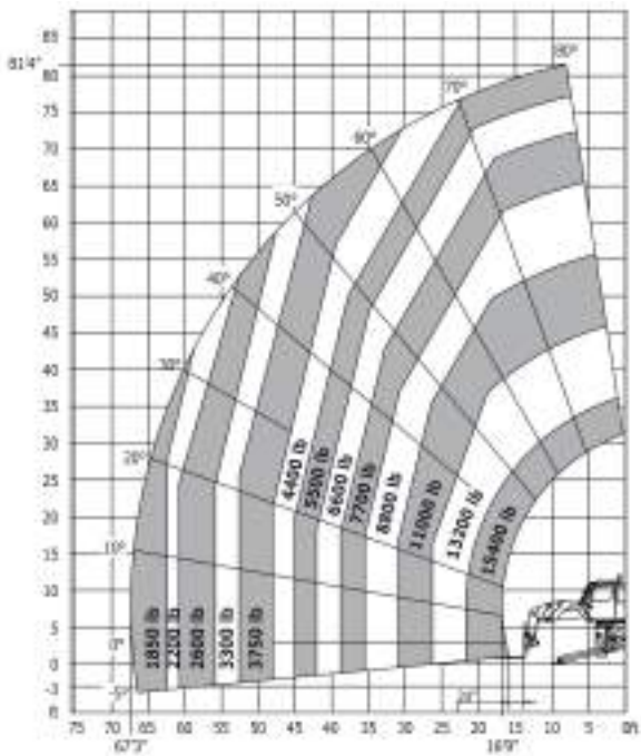
Rotación sobre estabilizadores en posición baja con horquillas
