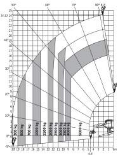
Rotación sobre estabilizadores en posición baja con cabestrante 5.000 kg
